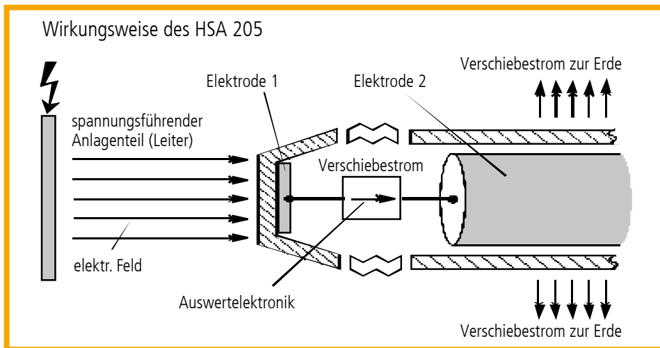
Bild 4 Funktionsprinzip
